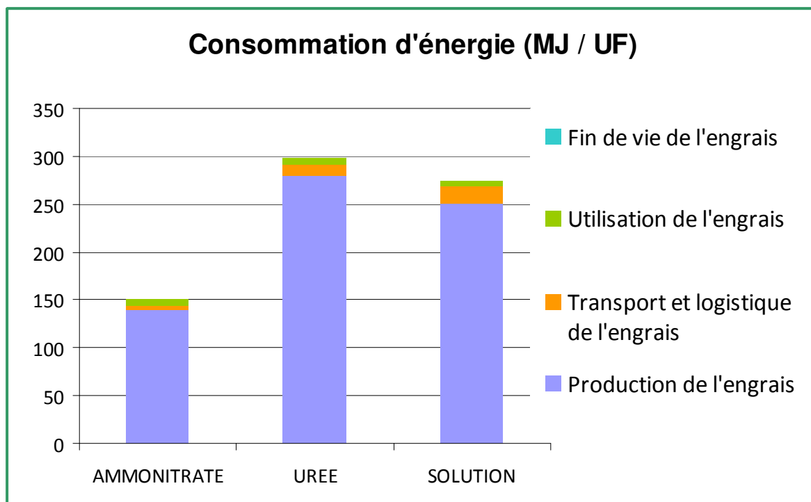
Figure 6 : Résultats de l'ACV comparative des trois formes pour l'indicateur de consommation d'énergie
